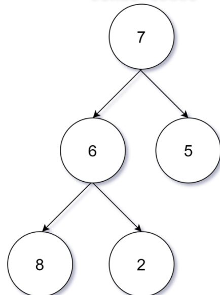
final tree1
