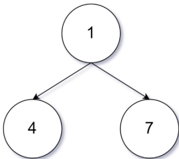
initial tree1
