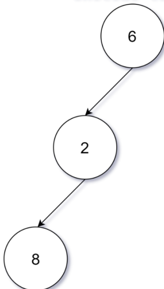
initial tree1
